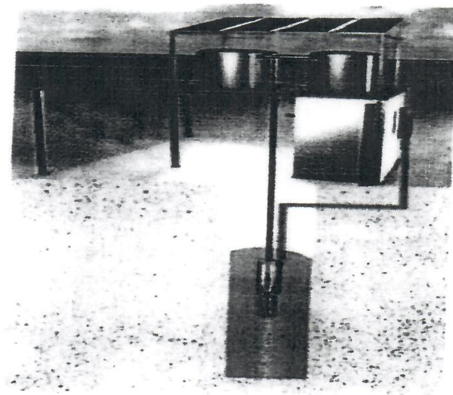
Modèle système forage d'eau avec pompe solaire
