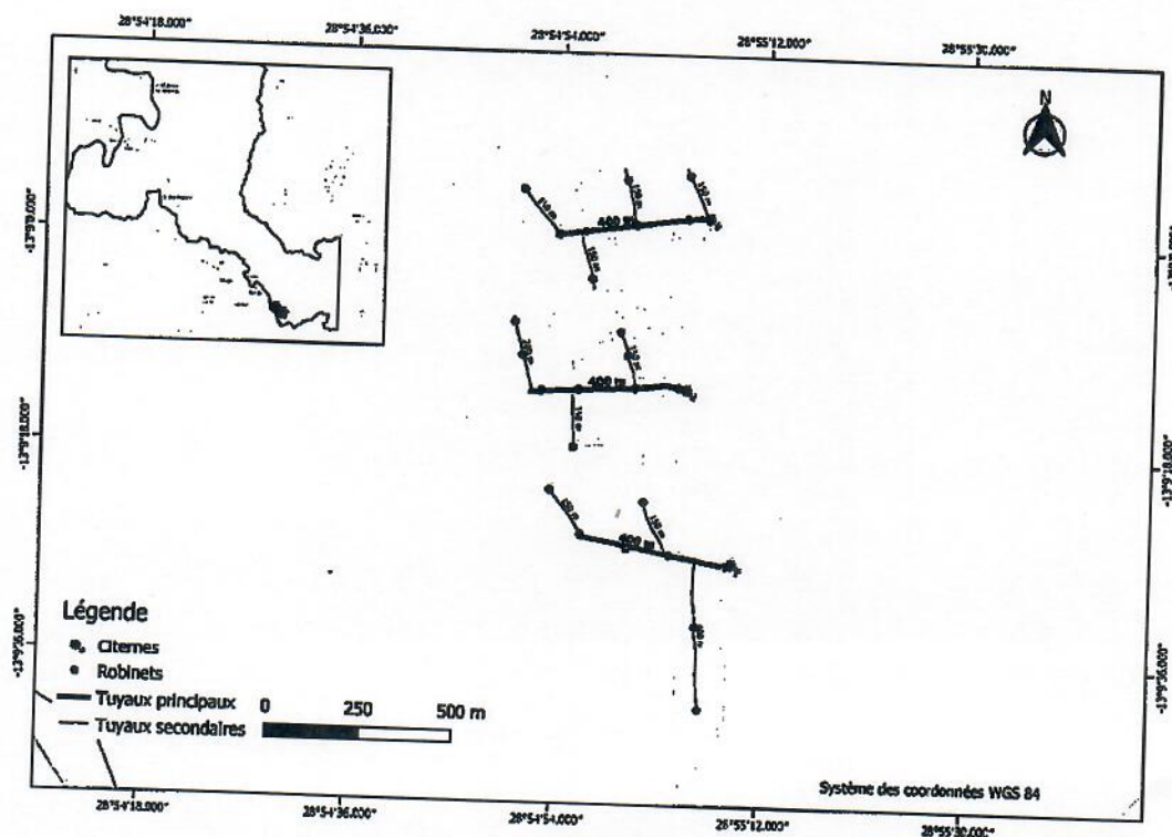
Figure 4. Schéma de distribution de l'eau dans le village Lonshi à partir des trois réservoirs existants.
